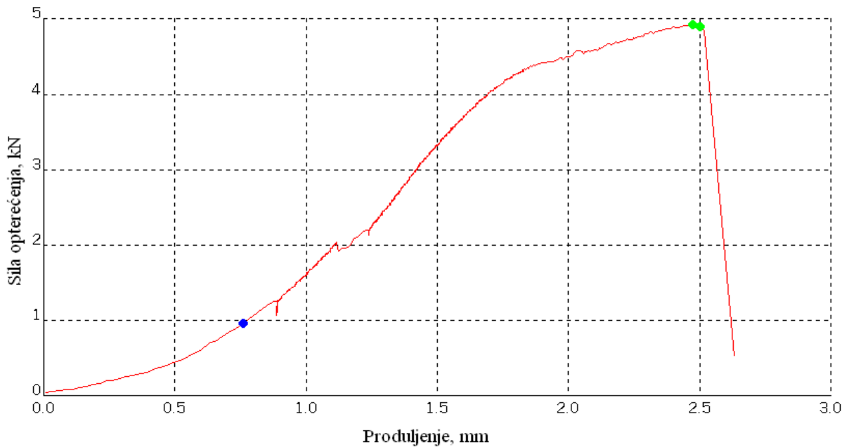
Slika 51. Ispitivanje uzorka 5
