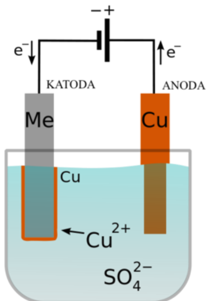
Slika 17. Shematski prikaz postupka galvanizacije [16]
