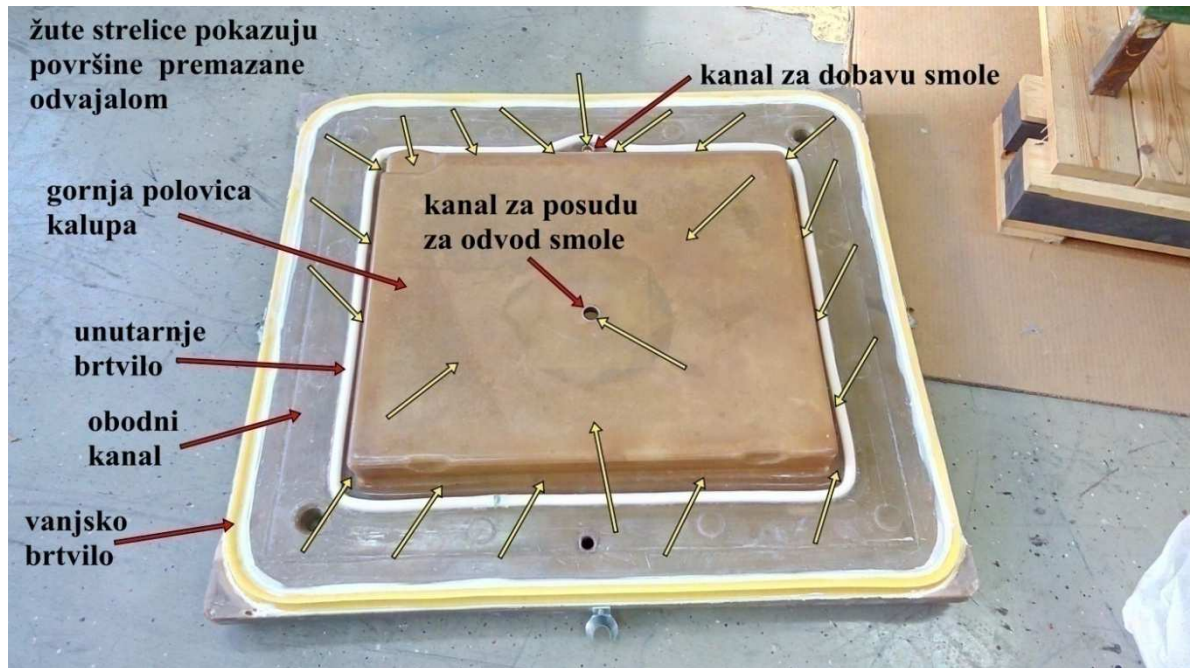
Slika 4.7. Gornja polovica kalupa: mjesta i površine premazane odvjalom
