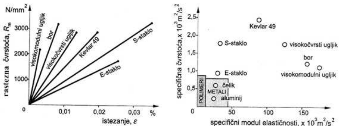
Slika 2.16. Svojtva vlakana: (a) krivulja "naprezanje-istezanje", (b) usporedba specifične čvrstoće i specifičnog modula elastičnosti metala i nekih vlakana [2]
