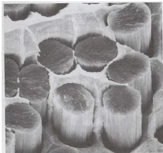
Slika 2.12. Legura Ag-Cu ojačana s ugljičnim vlaknima [4]
