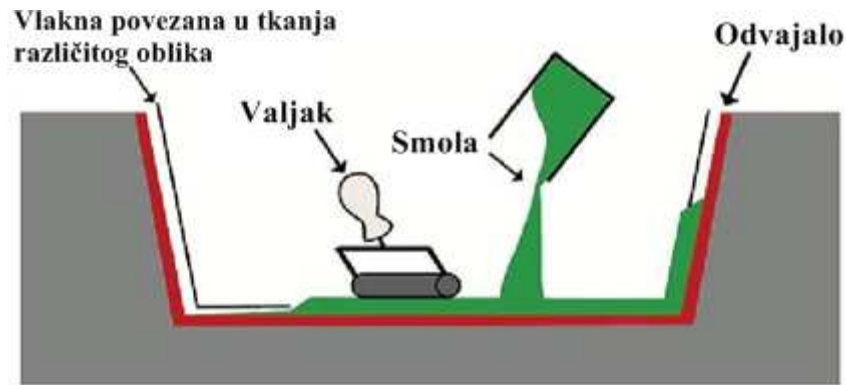
Slika 2.21. Proizvodnja kompozita laminiranjem [6]
