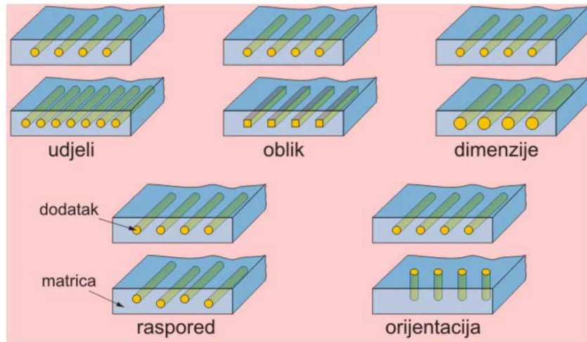
Slika 2.1. Faktori koji utječu na svojstva kompozita[4]
