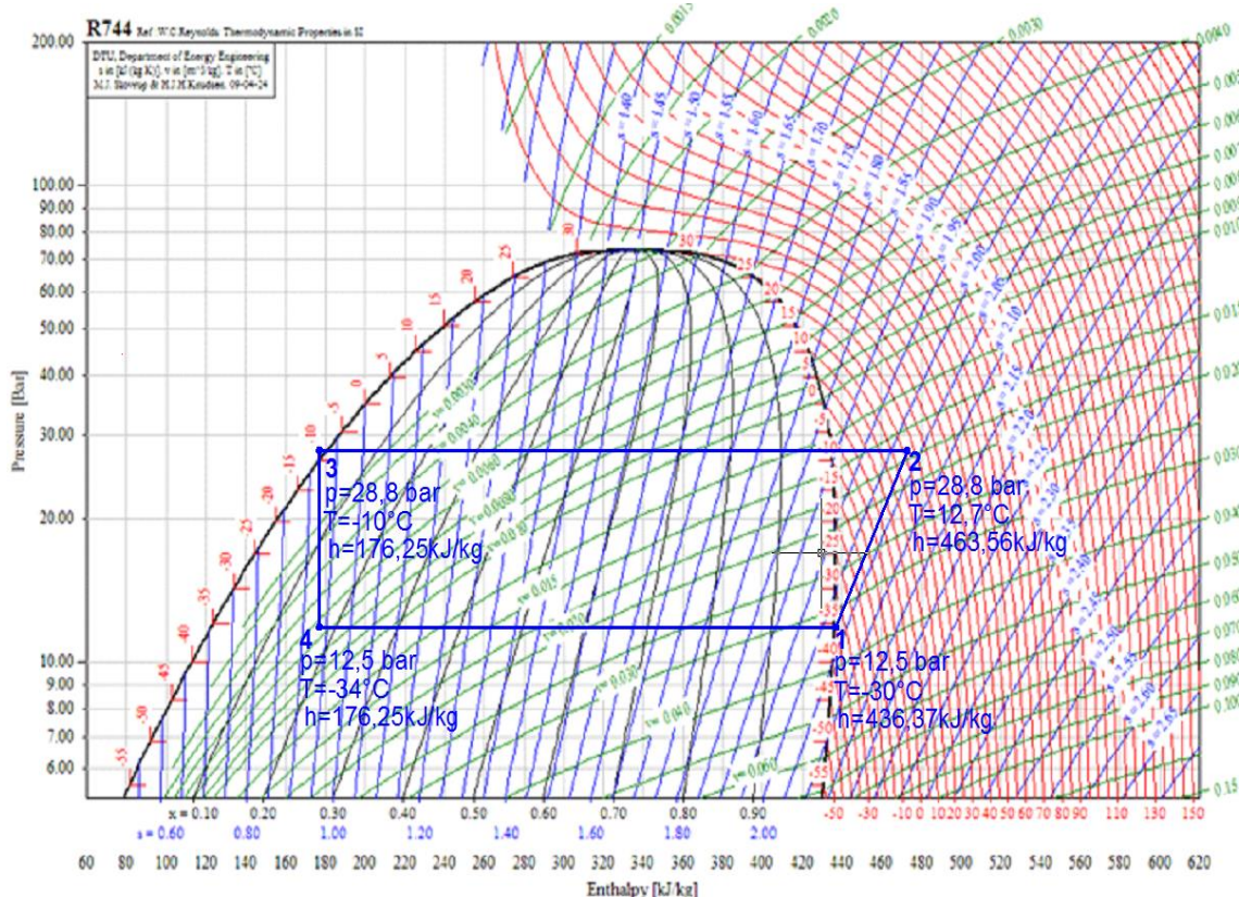
Dijagram 9. Rashladni proces u log p-h dijagramu za radnu tvar R744
