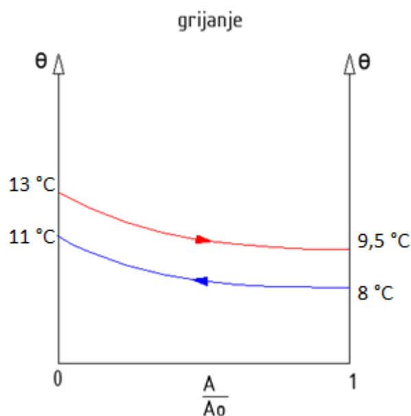
Slika 5.9. Dijagram međuzmjenjivača u režimu grijanja
