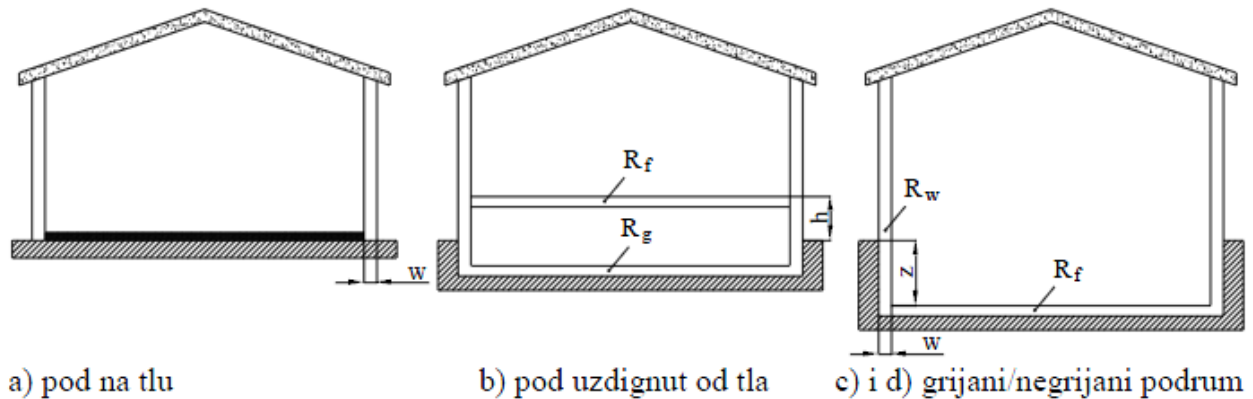
Slika 4.1. Različite izvedbe poda [12]
