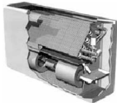
Slika 2.15. Ventilokonvektor u presjeku – zidna izvedba [3]
