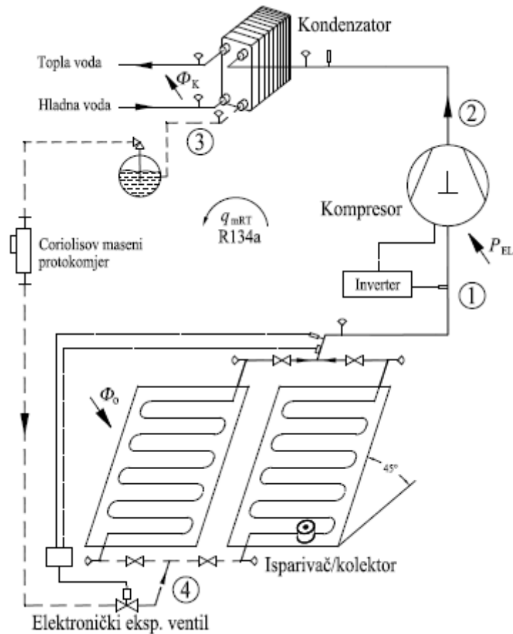
Slika 2.8. Shematski prikaz solarne dizalice topline [3]
