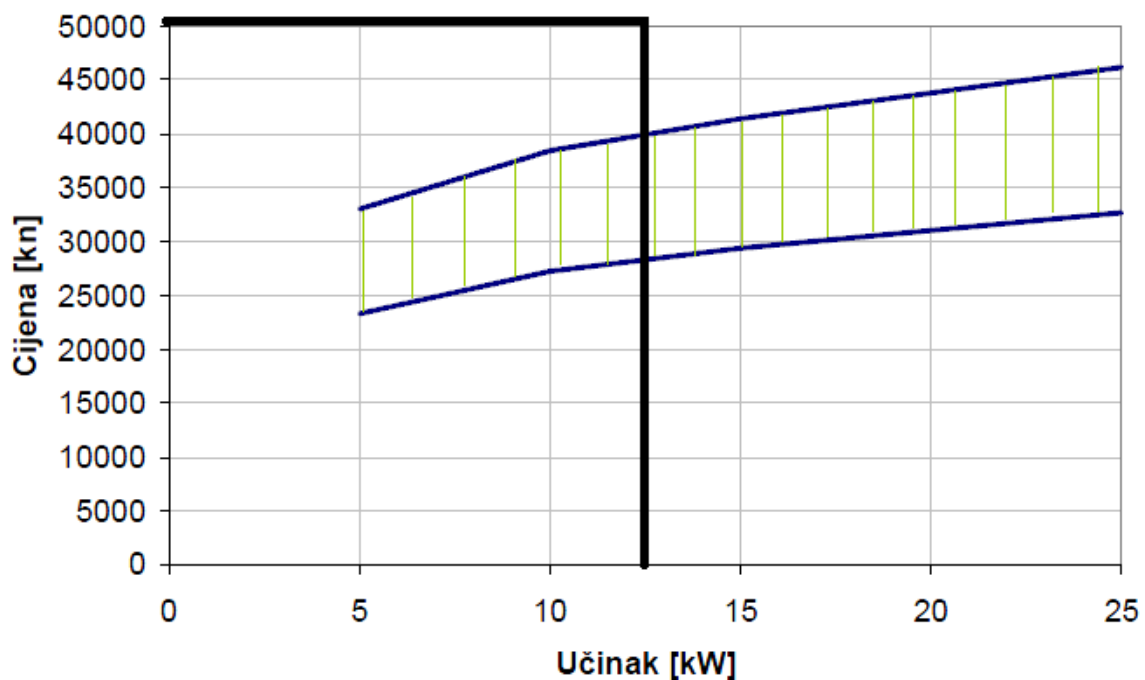
Slika 7.1. Cijena bunara i razvoda vode do dizalnice topline u ovisnosti o učinku [20]
