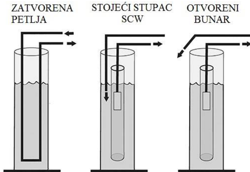
Slika 2.11. Usporedba različitih izvedbi izvora topline iz podzemne vode [5]
