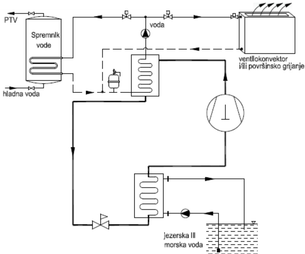
Slika 2.9. Dizalica topline voda-voda [3]
