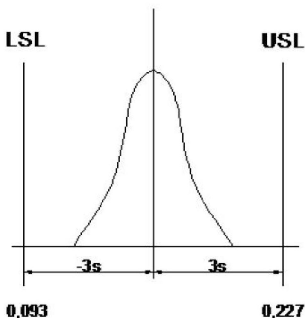
Slika 27. Granice tolerancije [8]
