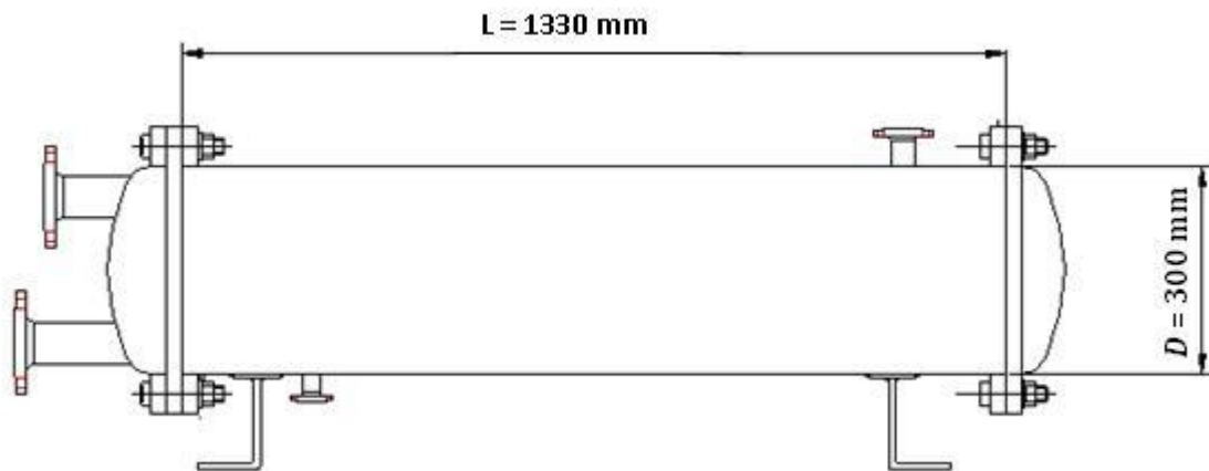
Slika 20. Dimenzije kondenzatora
