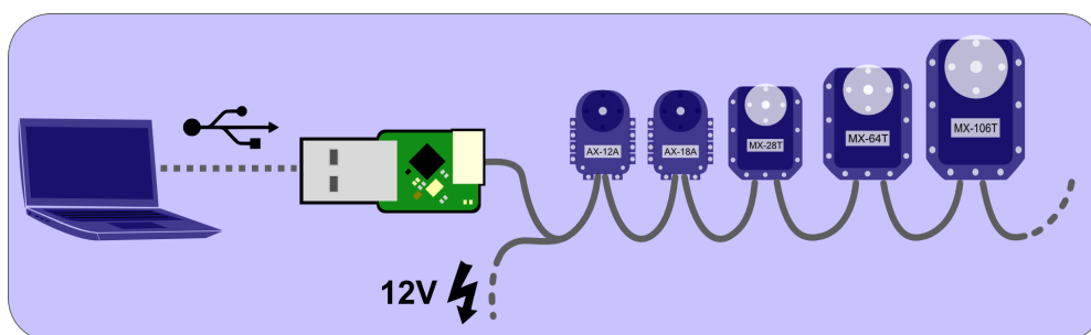
Slika 79: Shematski prikaz spoja USB2AX i servo motora
