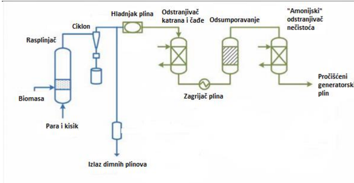
Slika 13. Shema pročišćavanja generatorskog plina [9]
