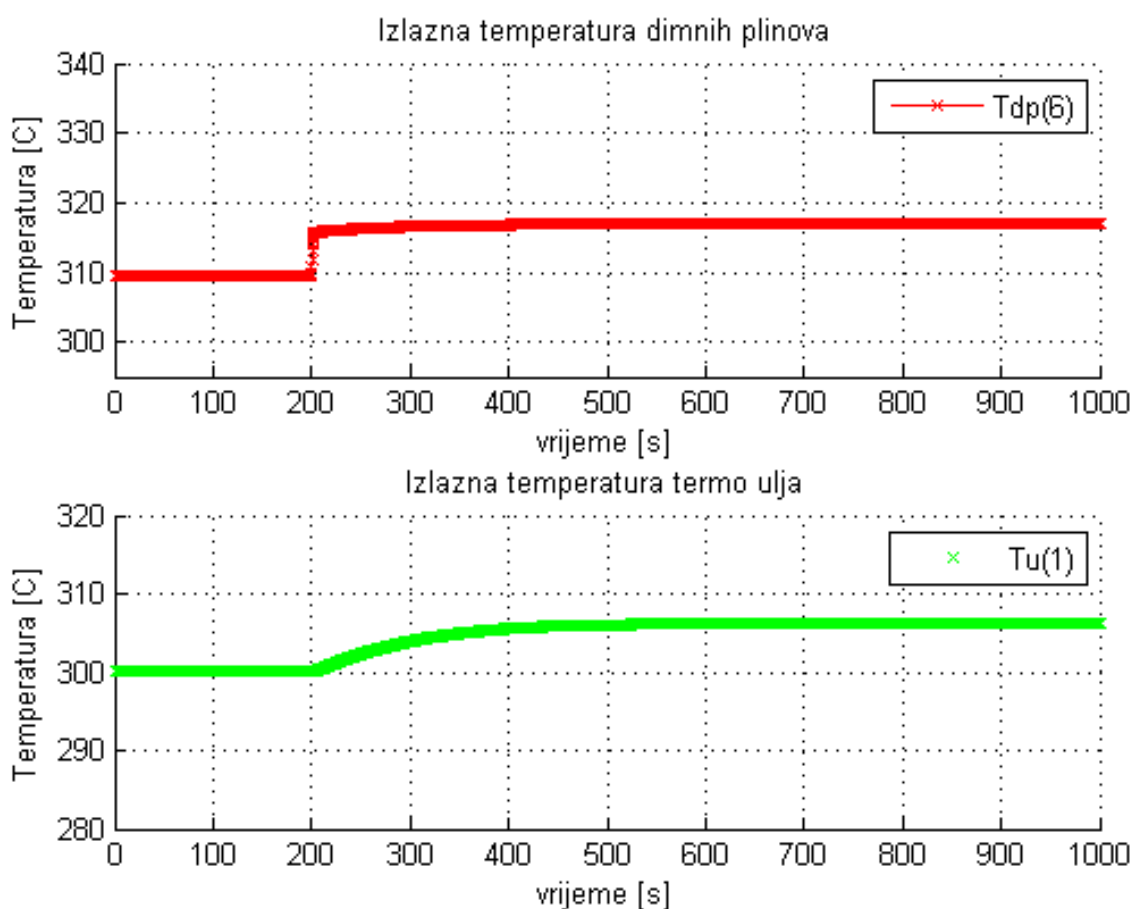
Slika 33. Odzivi na poremećaj ulazne temperature dimnih plinova
