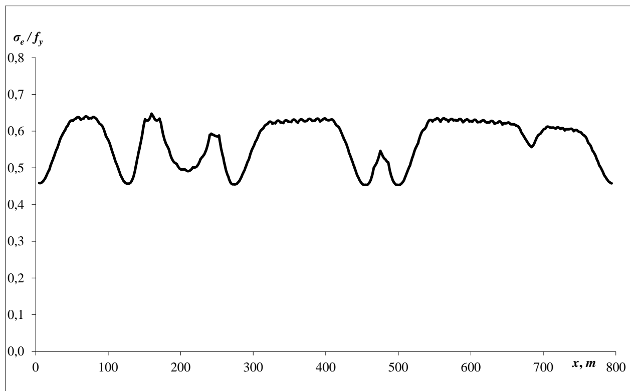
Slika 17. Omjer ekvivalentnog i dozvoljenog naprezanja po duljini cjevovoda
