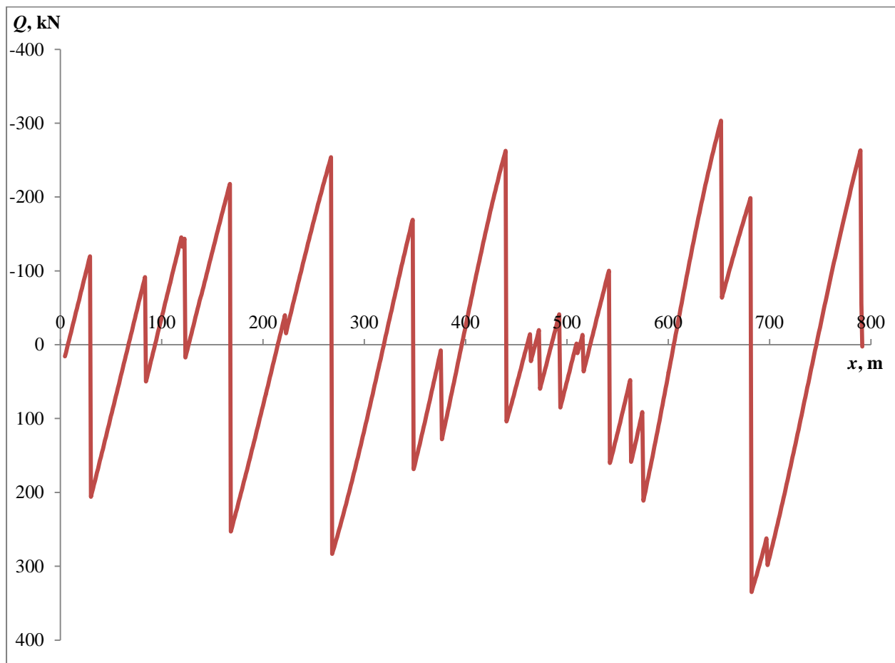
Slika 18. Smična sila za originalni profil
