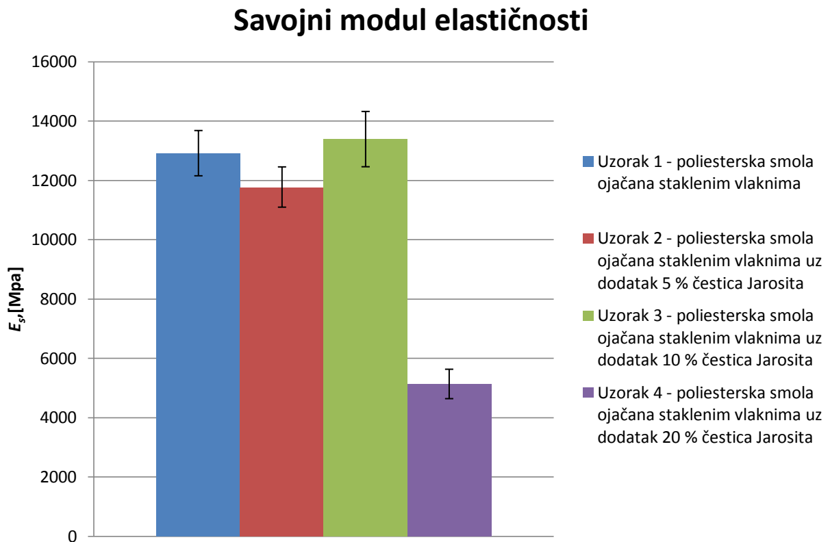
Slika 26. Usporedba vrijednosti savojnog modula elastičnosti uzoraka bez i sa česticama jarosita kao punila u poliesterskom kompozitu
