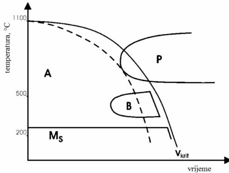
Slika 3.2. TTT dijagram s ucrtanim krivuljama hlađenja; A ... austenit; B ... bainit; P ... perlit; M_s ... martenzit [9]
