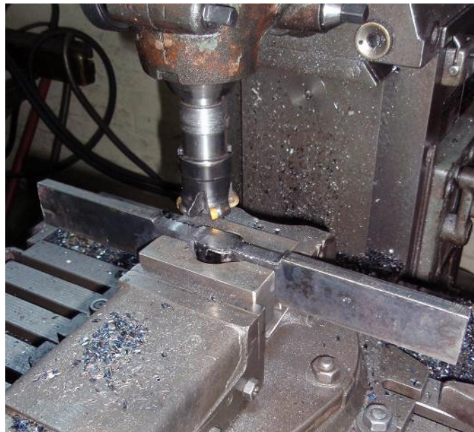
Slika 5.15. Glodanje epruvete za statički vlačni pokus
