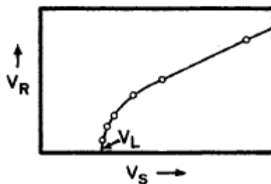
Slika 26. Metoda rezidualne brzine [19]
