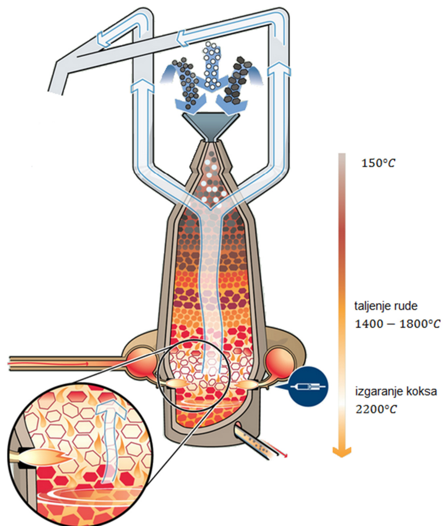
Slika 2. Visoka peć [4]
