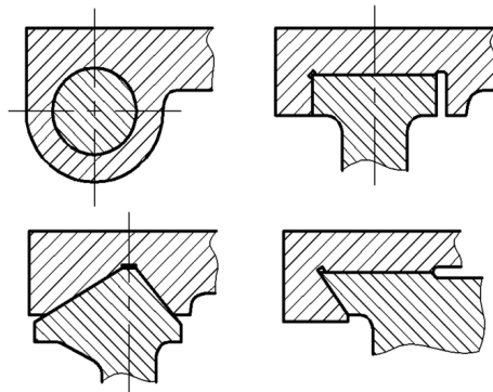
Slika 24. Oblici hidrodinamskih kliznica [6]
