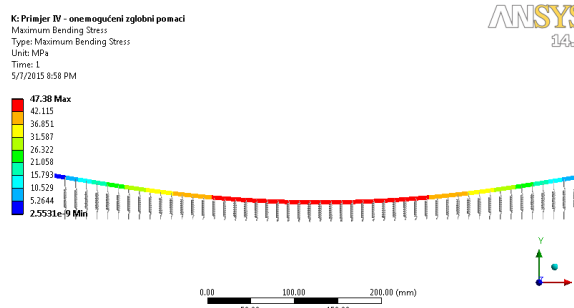
Slika 56. Raspodjela savojnog naprezanja
