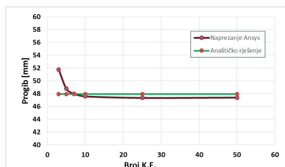
Slika 57. Konvergencija progiba i savojnog naprezanja za 1-D ANSYS model
