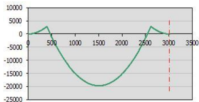
Slika 40. Momentni dijagram
