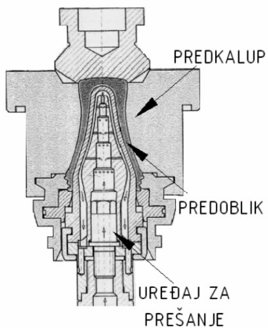
Slika 47. Prešnjem se postiže predoblik[14]
