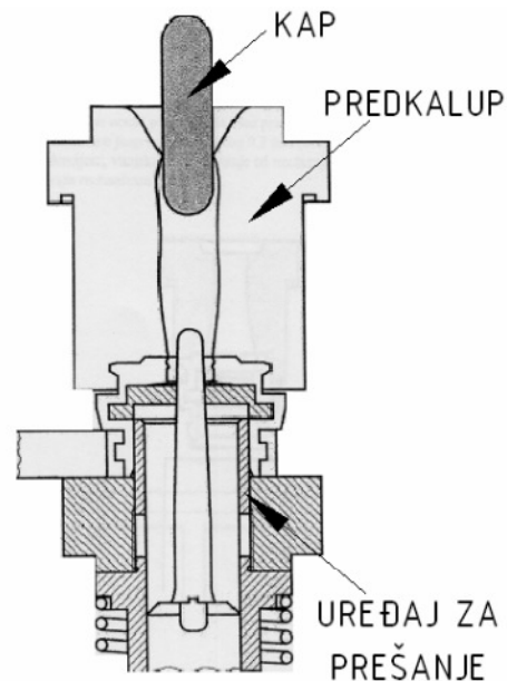
Slika 51. Kap ulazi u predkalup[14]
