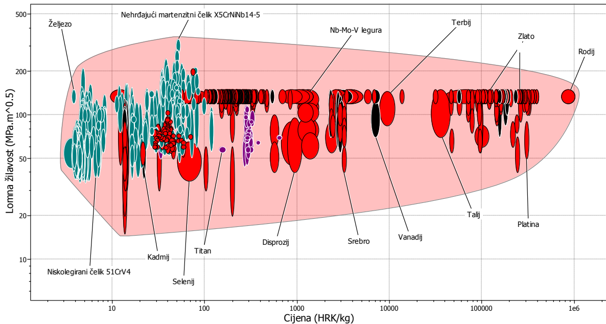
Slika 24. Dijagram cijena- lomna žilavost materijala koji su prošli osnovni kriterij u Ces EduPack-u 2009 na razini 3 [10]
