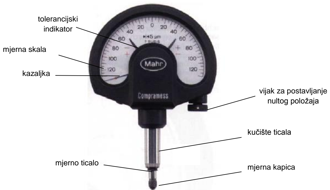
Slika 44. Sastavni dijelovi komparatora [7]
