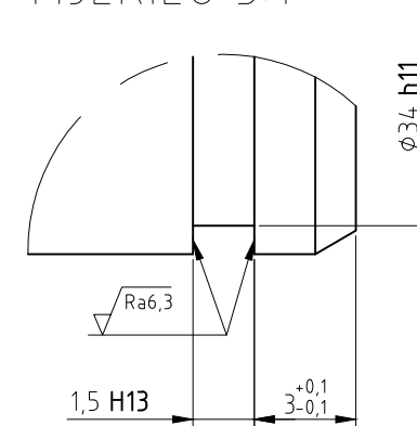
DETALJ C-C MJERILO 5:1
