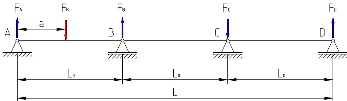
Slika 9. Nosač vozne staze na četiri oslonca
