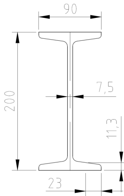
Slika 11. Dimenzije profila I 200
