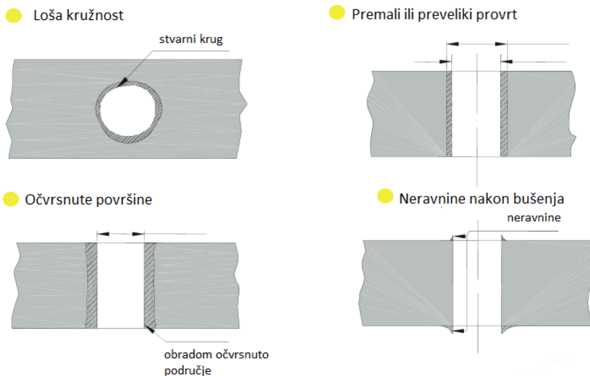
Slika 49. Greške početnog provrta [21]
