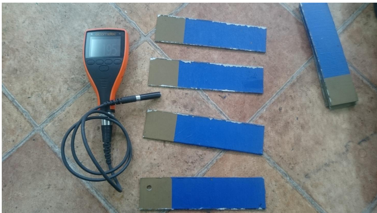
Slika 19. Uređaj Elcometer 456 za ispitivanje debljine suhog filma premaza i ispitni uzorci
