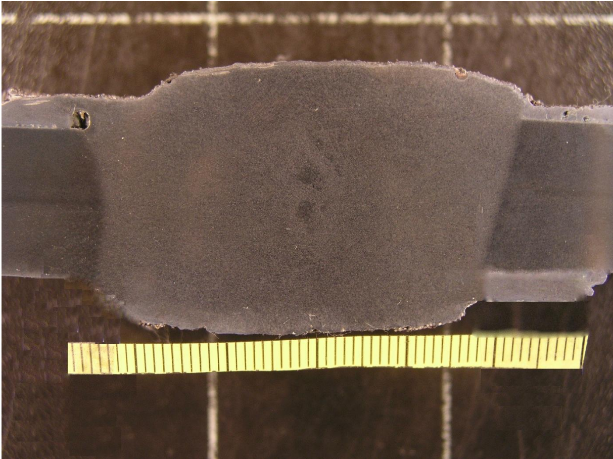
Slika 46 Makroizbrusak zavara
