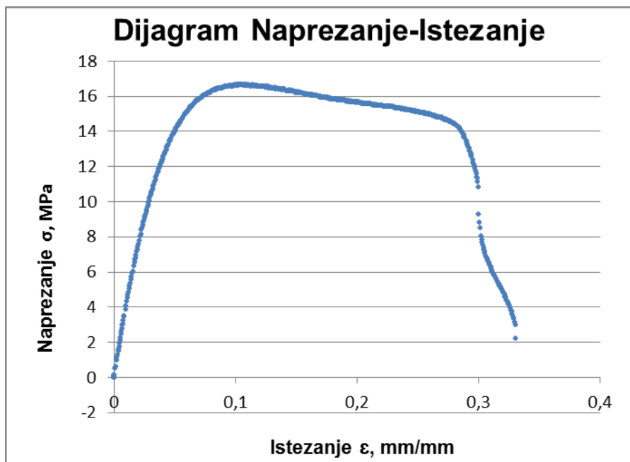
Slika 6.11. Dijagram Naprezanje-Istezanje za epruvetu nakon balističkog testa izrezanu iz ploče br. 1
