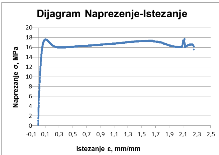
Slika 6.10. Dijagram Naprezanje-Istezanje za epruvetu prije balističkog testa izrezanu iz ploče br. 1
