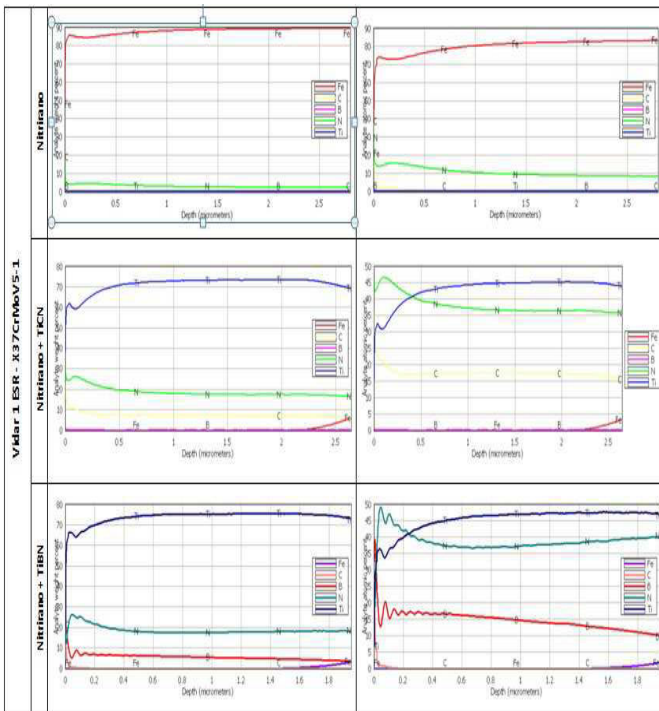
Slika 12. Rezultati GDOES analize različito površinski obrađenih uzoraka od čelika X37CrMoV5-1
