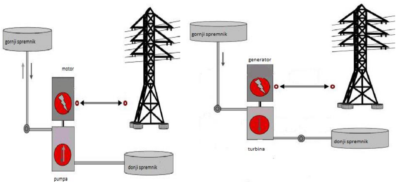
Slika 19. Shema tjeranja vode pumpom i puštanja vode na turbinu_2 [26]
