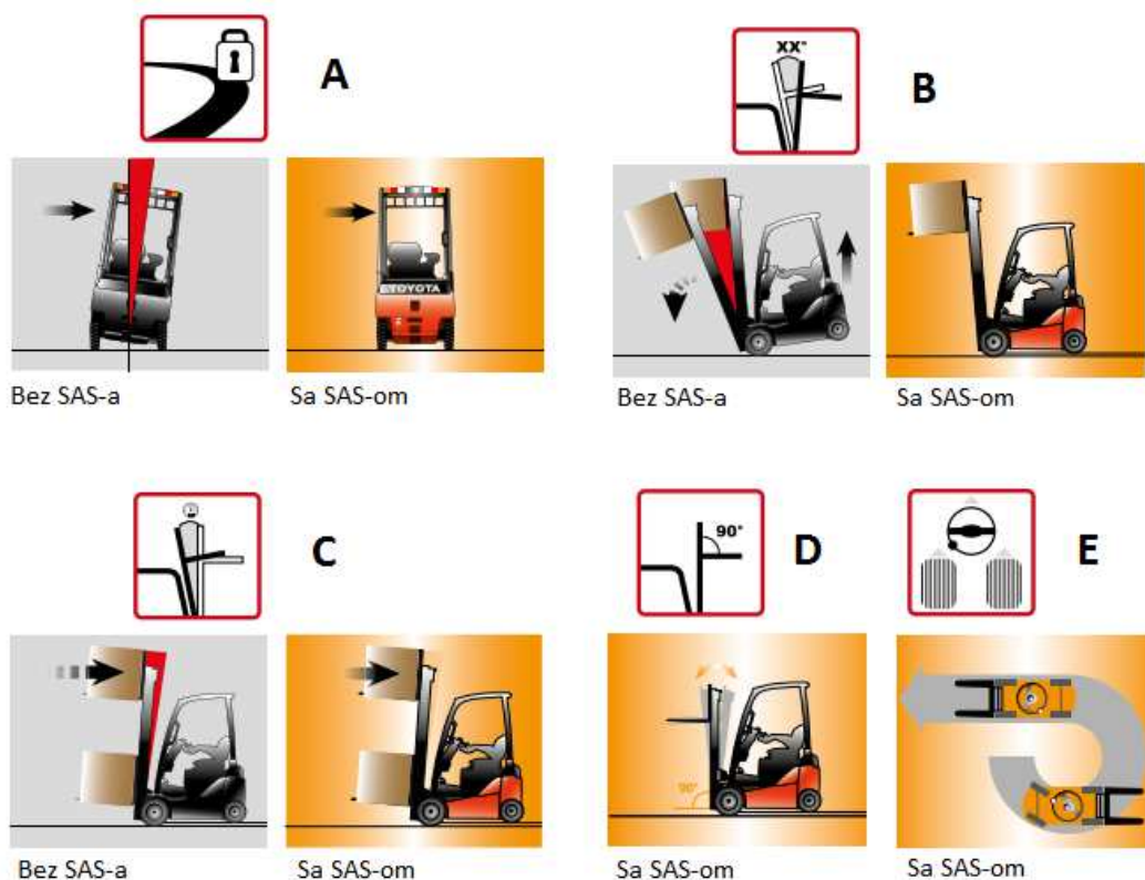
Slika 45. Funkcije Toyota "SAS" sustava [43]
