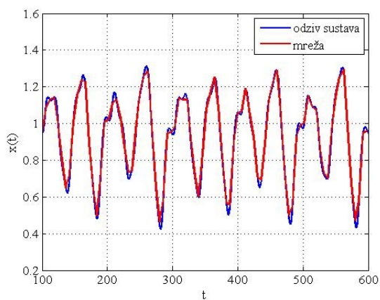
Slika 4.20. Učenje mreže s 12 neurona prvog sloja i 8 neurona drugog sloja
