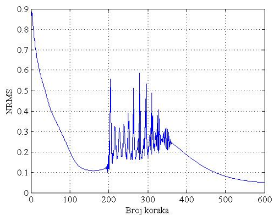
Slika 4.18. Učenje mreže s 8 neurona prvog sloja i 12 neurona drugog sloja
