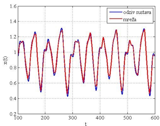
Slika 4.19. Učenje mreže s jednakim brojem neurona sakrivenih slojeva
