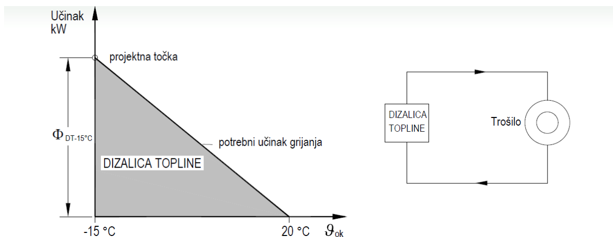
Slika 3. Monovalentni način rada dizalnice topline [3]
