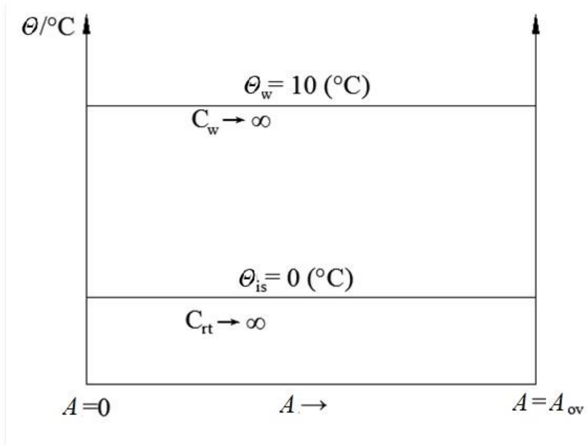
Slika 16. Prikaz temperaturne promjene struja u ovisnosti o površini isparivača
