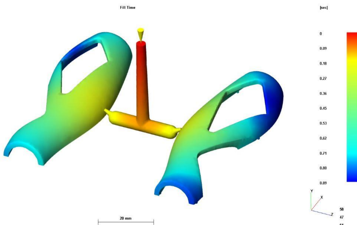
Slika 6.7. Vrijeme punjenja
