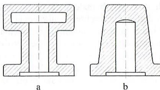
Slika 5.33. Proizvod s podrezanim vanjskim i unutarnjim plohama; b) Proizvod bez podrezanih ploha [10]
