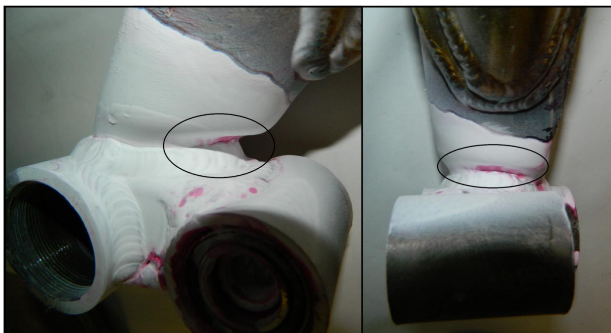
Slika 25. Indikacija pukotine
