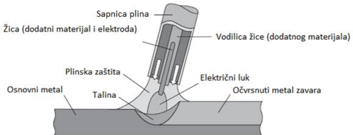
Slika 2. Shema MIG postupka zavarivanja [1]
