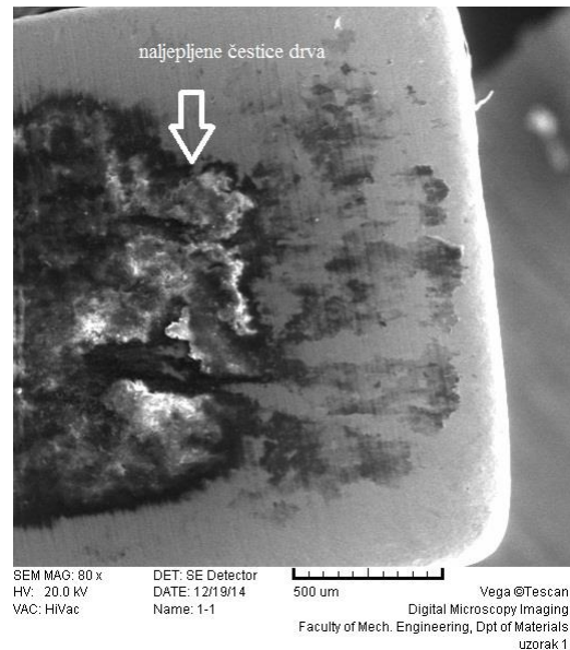
Slika 35. Naljepljivanje čestica drva na reznu površinu uzorka 1
