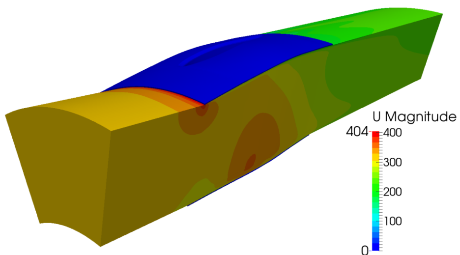
Slika 16 Polje brzine po volumenu
