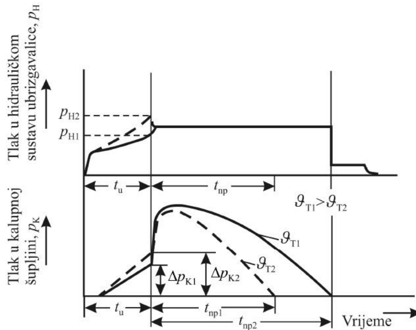
Slika 2.6. Utjecaj temperature taljevine na tijek tlaka u hidrauličkom sustavu ubrizgavalice i kalupnoj šupljini: \vartheta_T - temperatura taljevine, t_u - vrijeme ubrizgavanja [5]
