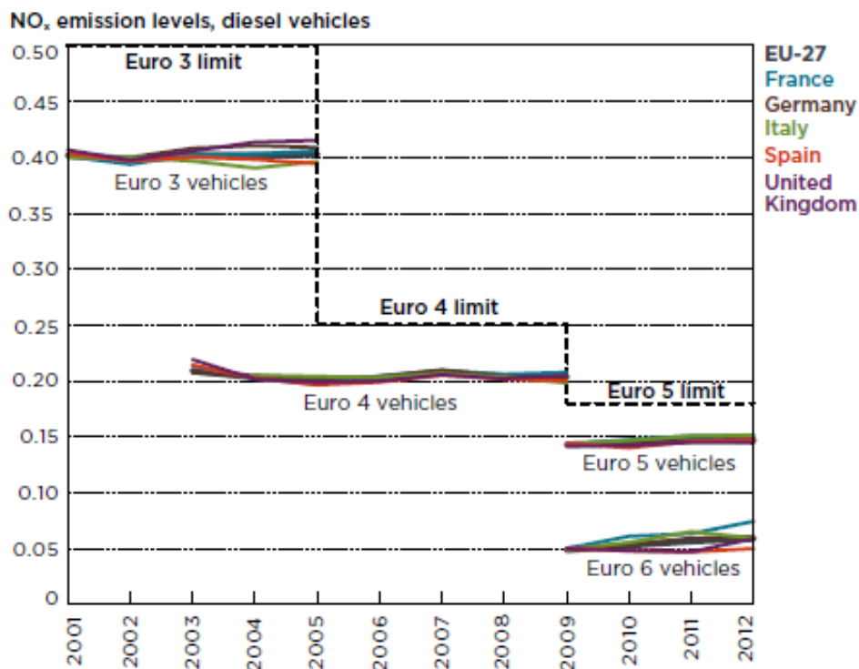
Slika 7.3. Razina emisija NO x osobnih vozila pogonjenih Dieselovim motorom prema državama [21]
