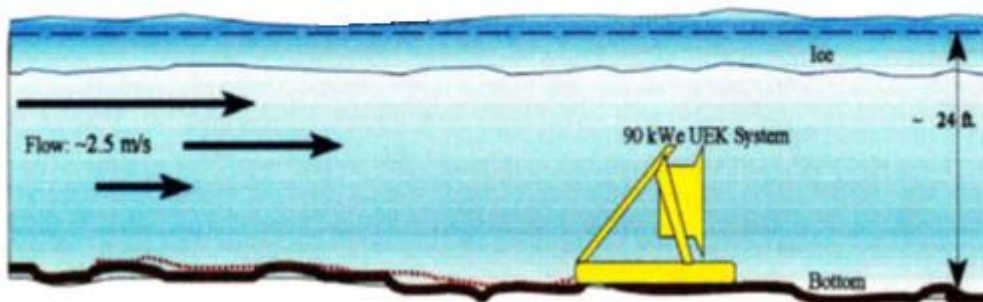
Slika 17. Pričvršćivanje na morsko ili riječno dno gravitacijom
