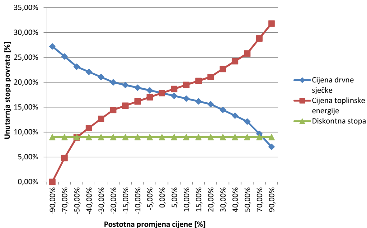
Slika 30. Utjecaj promjene cijene toplinske energije i cijene drvne sječke na IRR postrojenja na biomasu
