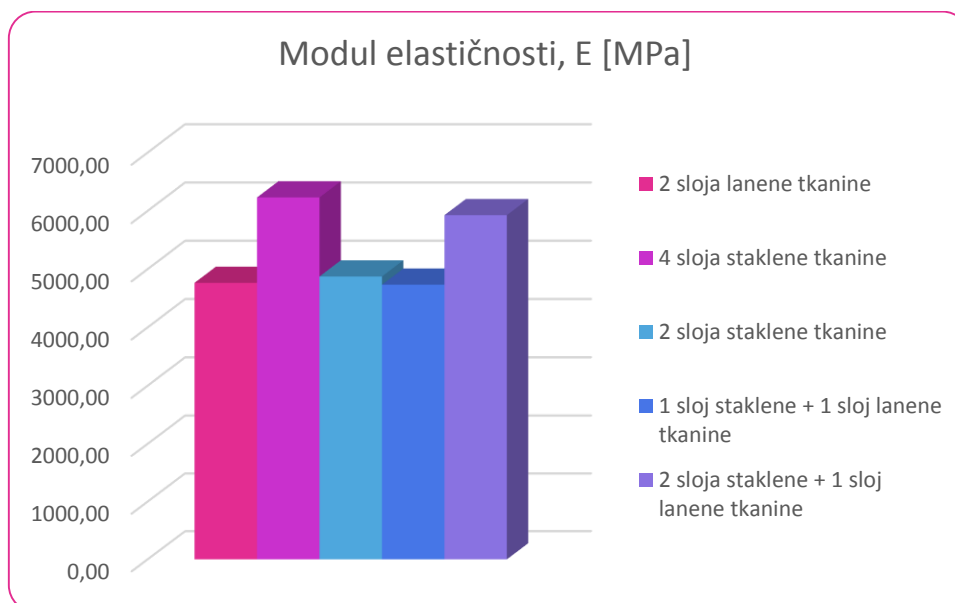
Slika 57. Usporedba uzoraka prema modulu elastičnosti
