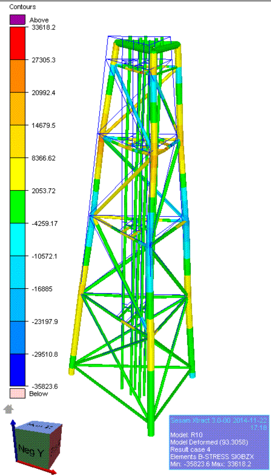
Slika 32. Naprezanje zbog savijanja \sigma_{zx} [ kN/m^2 ] slučaj opterećenja 4 ( H = 7.90\ m, T = 6.06\ s, \beta = 90^\circ .)
