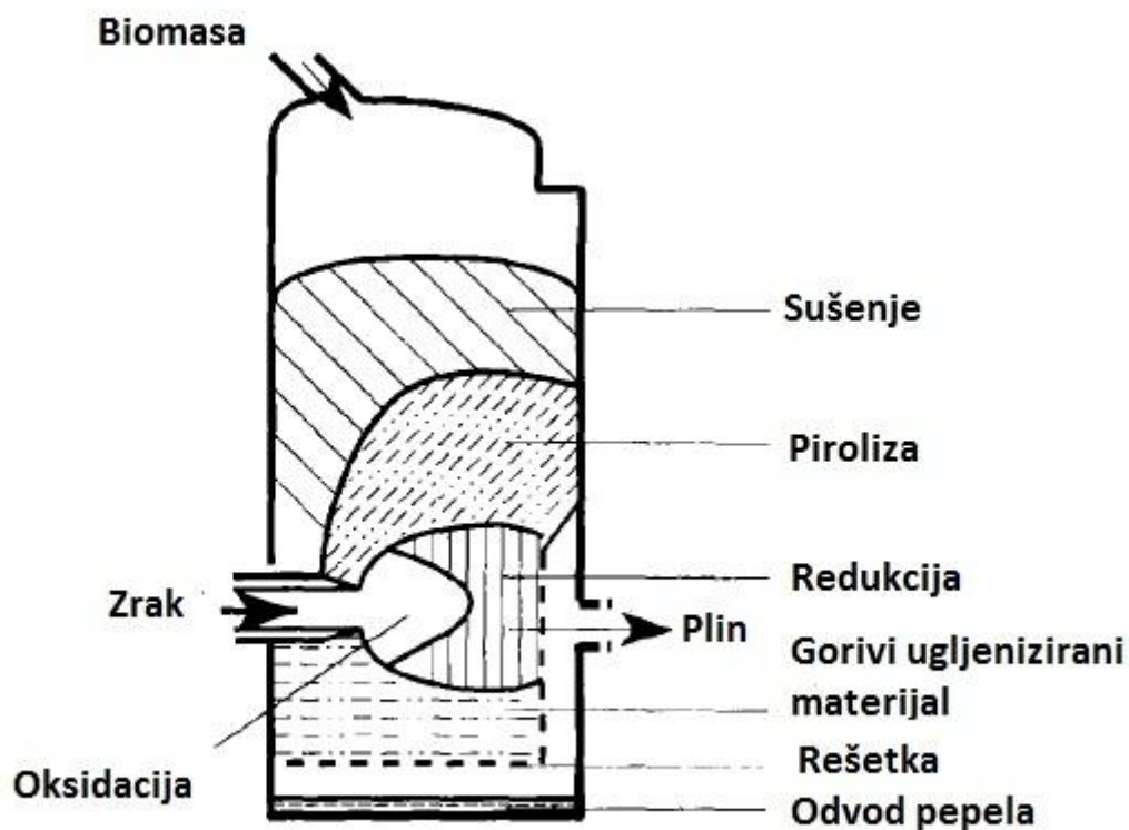
Slika 9. Križni reaktor [4]
