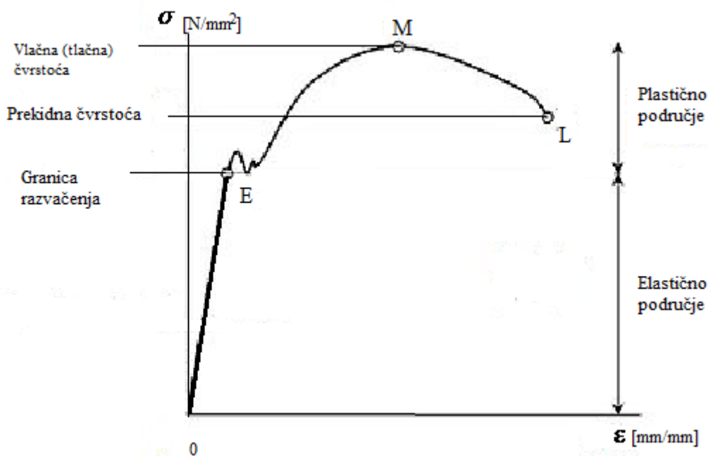
Slika 12. Dijagram naprezanja-istezanja
