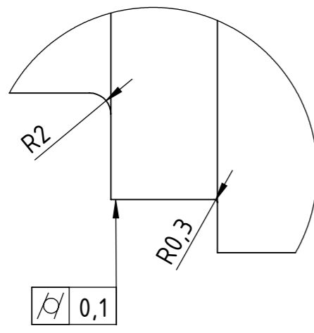
DETALJ A 2 : 1
