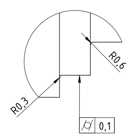
DETALJ B 2 : 1
