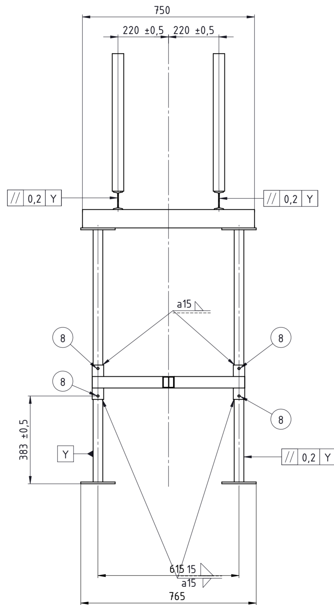
PRESJEK A-A 1 : 10
