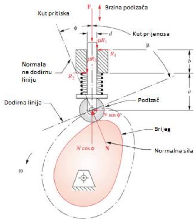
Slika 7.2 Trenutak maksimalnog kuta pritiska \phi za brijeg općenito
