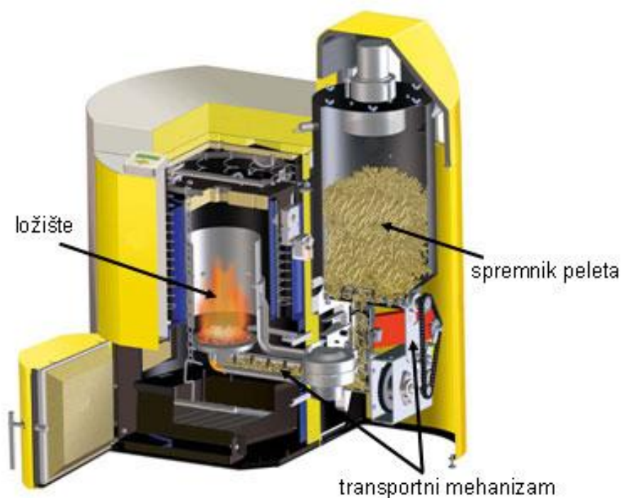
Slika 3: Peć na pelete [20]
