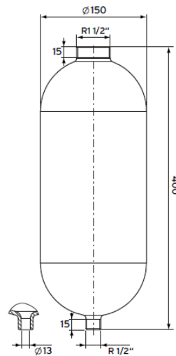
Slika 4.2 Kompenzacijska posuda
