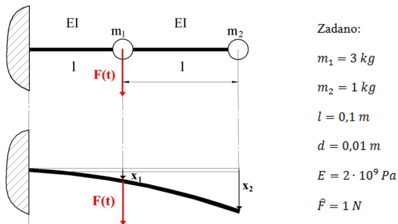
Slika 34 - Fleksijski vibracijski sistem s 2 stupnja slobode gibanja
