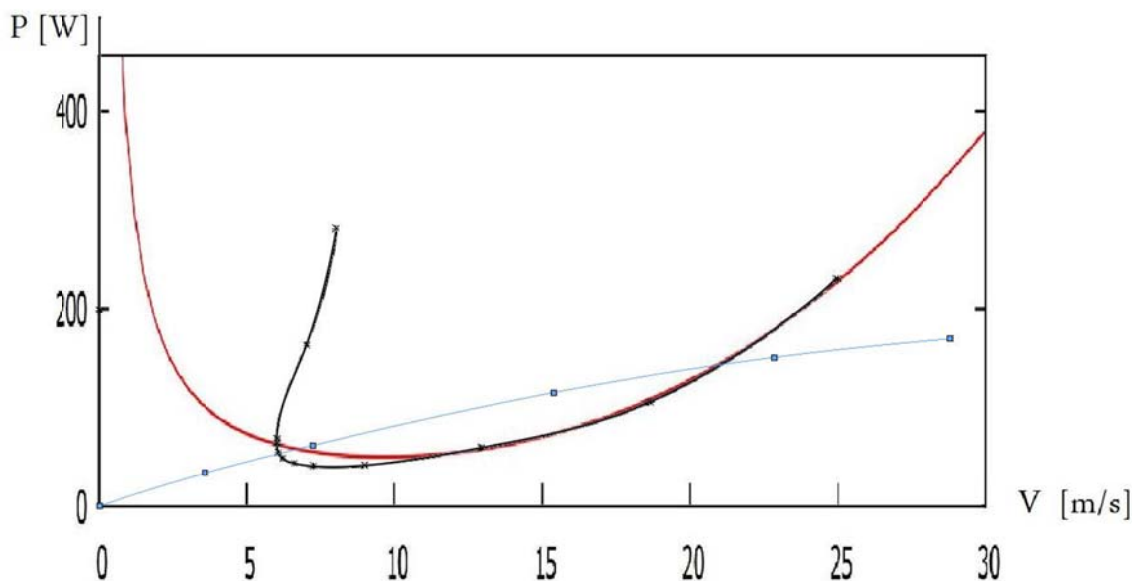
Slika 27: Dijagram potrebne snage za horizontalni let po Leishmanu (cveno), teoriji otpora (crno) i eksperimentalna raspoloživa snaga (plavo) u ovisnosti o brzini leta
