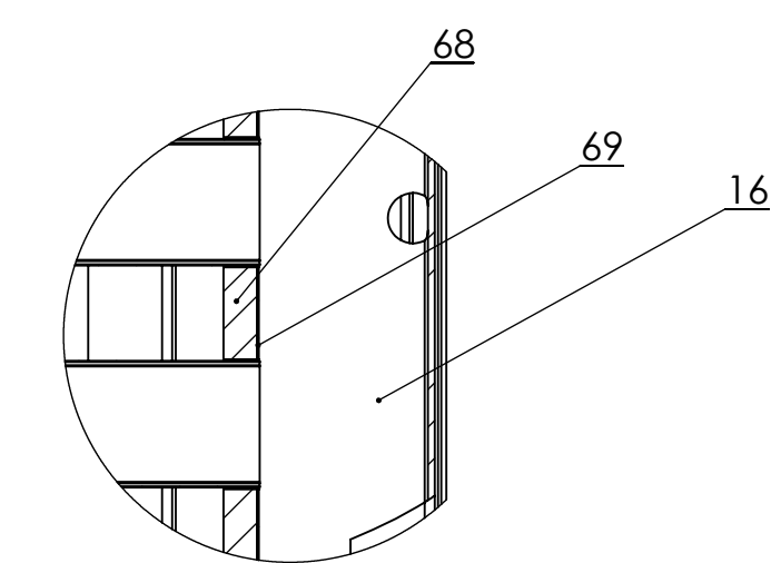
DETALJ A M1:5
