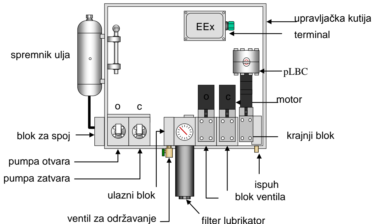
Slika 11. Grafički prikaz upravljačkog uređaja
