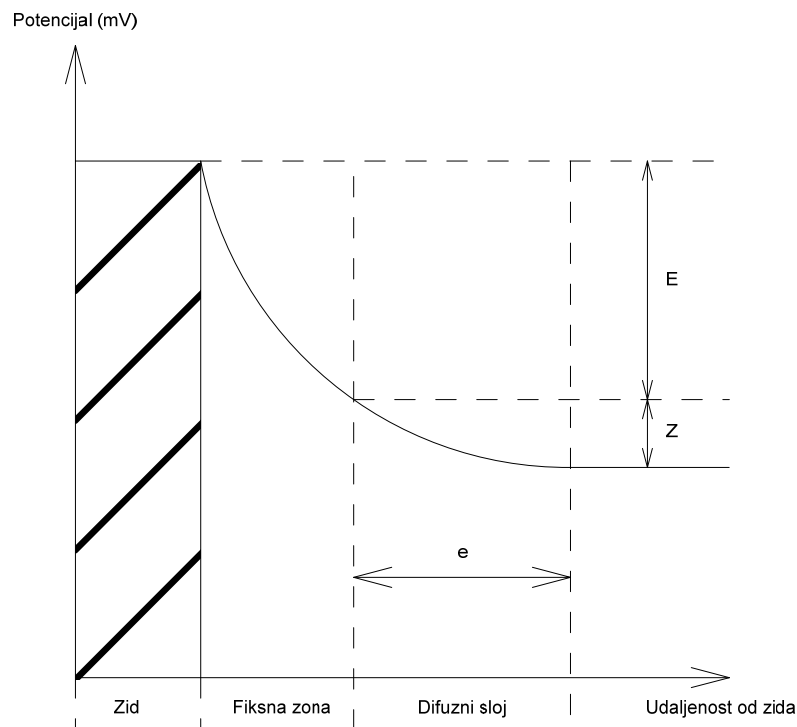
Slika 1. Zeta potencijal
