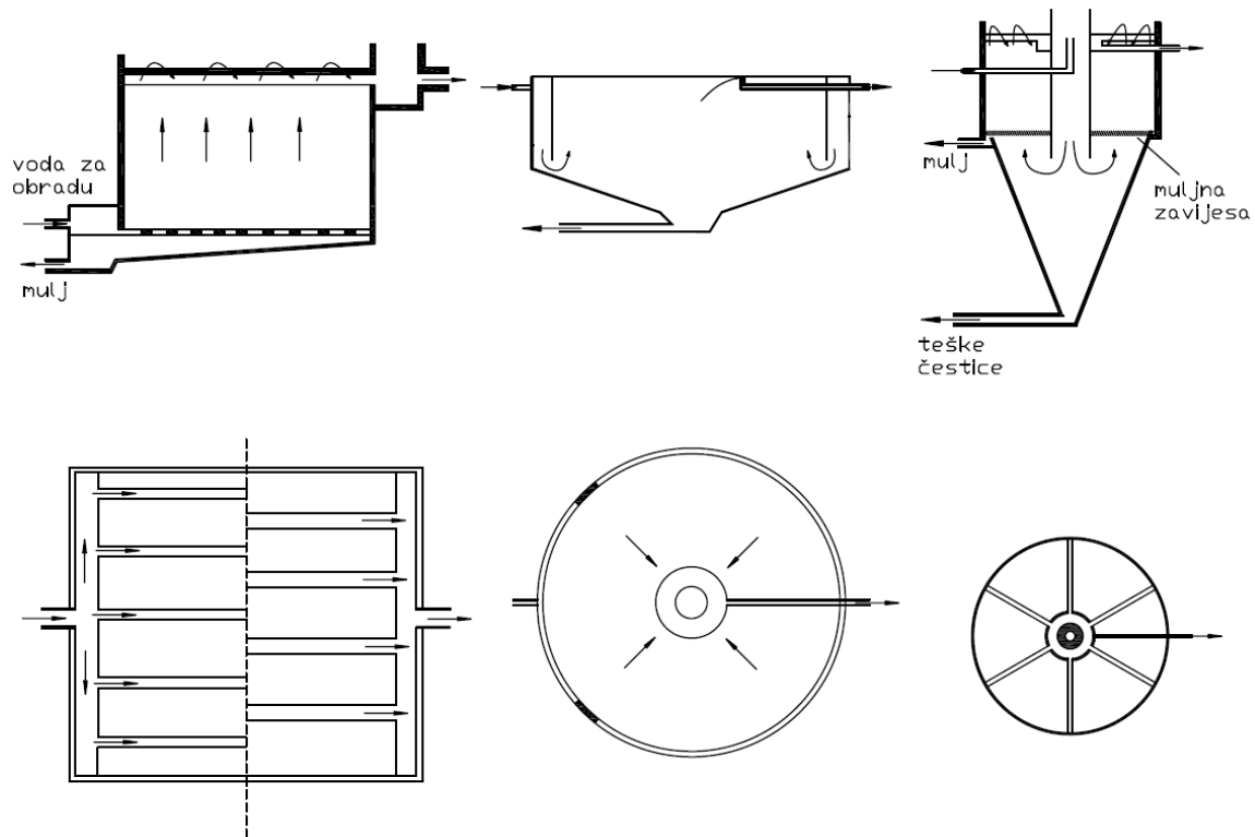
Slika 9. Vertikalni taložnici
