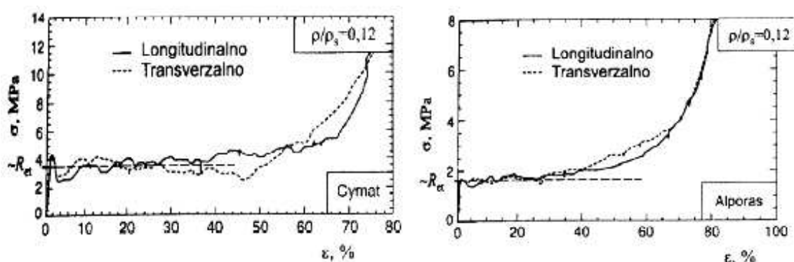
Slika 3.1. Dijagrami “naprežanje-skraćenje” metalnih pjena pri tlačnom opterećenju /12/
