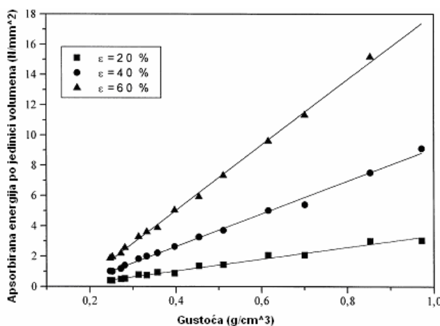
Slika 6.2. Dijagram apsorbirane energije udara po jedinici volumena AlSi 4 pjena različitih gustoća pri tlačnoj deformaciji od \varepsilon = 20\% , 30\% , 40\% i 60\% /28/
