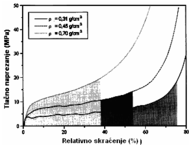
Slika 6.3. Tlačna karakteristika AlSi12 metalne pjene različitih gustoća /28/
